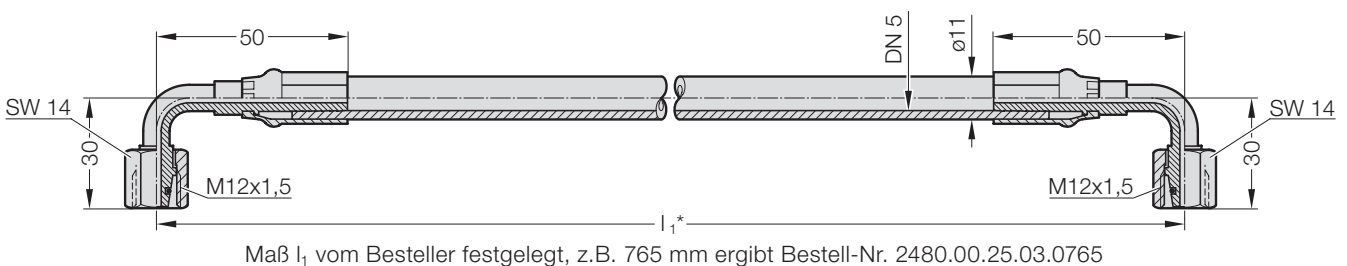
2480.00.25.03. Schlauch – Dichtkegel mit Überwurfmutter und O-Ring (90° abgewinkelt/beidseitig)
