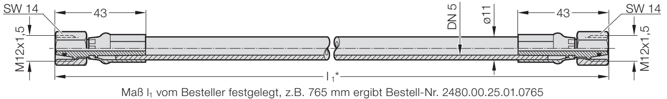
2480.00.25.01. Schlauch – Dichtkegel mit Überwurfmutter und O-Ring (gerade/gerade)
