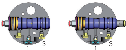
Patronenventil Standard 2489.14.1001 Patronenventil Gaskühlung 2489.14.1001. .N
