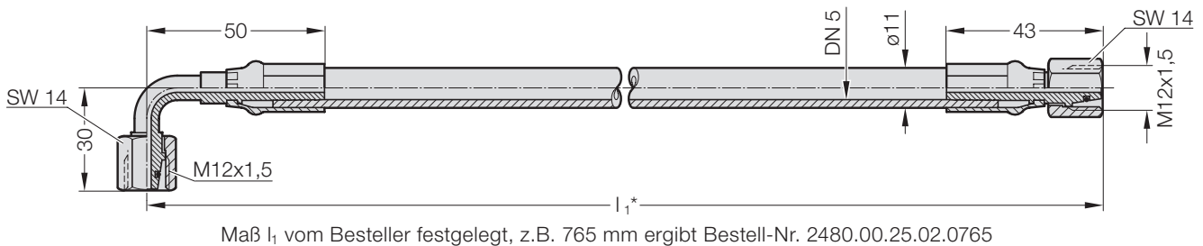
2480.00.25.02. Schlauch – Dichtkegel mit Überwurfmutter und O-Ring (90° abgewinkelt/gerade)
