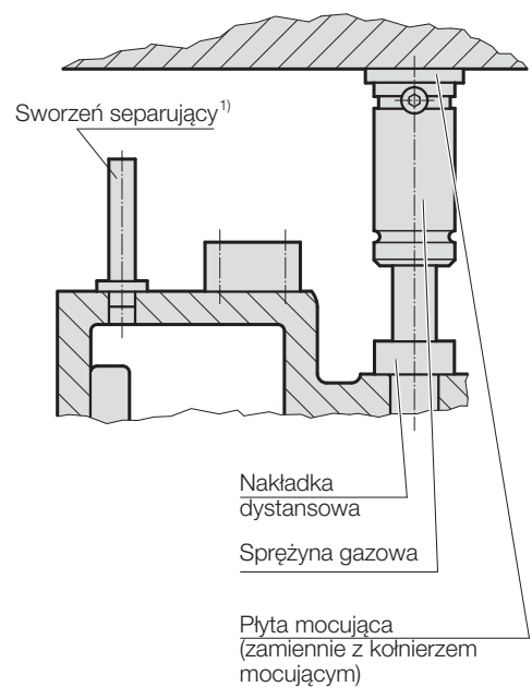
Przykład 2: Zastosowanie sprężyny gazowej zamocowanej w części górnej
