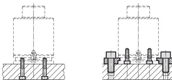
z dolną płytą-adapterem
