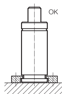
Mocowanie za pomocą 2480.007./008.
