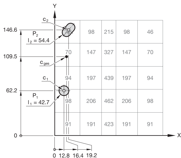
Immagine 23: Modello di foro eccentrico
