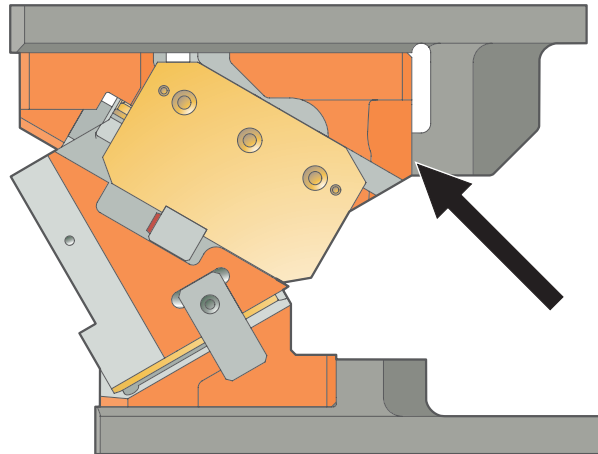
Immagine 2: Basamento del cursore con spallamento superiore
