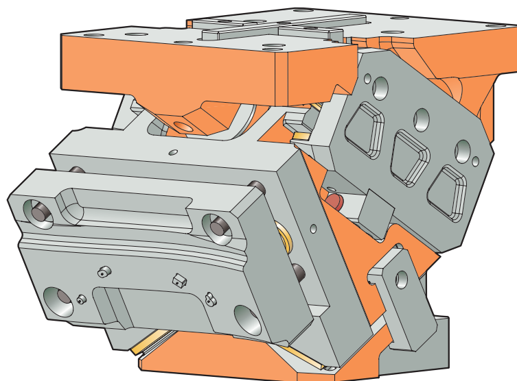
Immagine 8: Cursore con piastra raschiatore
