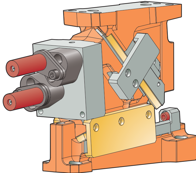
Immagine 7: Cursore con raschiatore elastomerico
