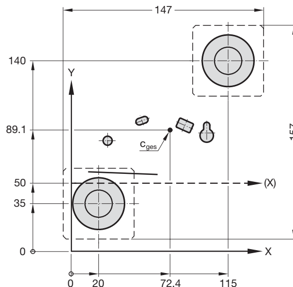
Immagine 16: Modello di foro con piastra di raschiatura
