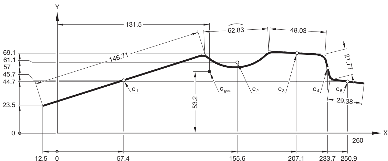
Immagine 11: Contorno di taglio approssimato
