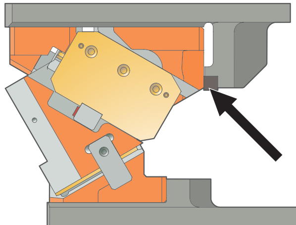
Immagine 3: Basamento del cursore con spallamento superiore con cuneo
