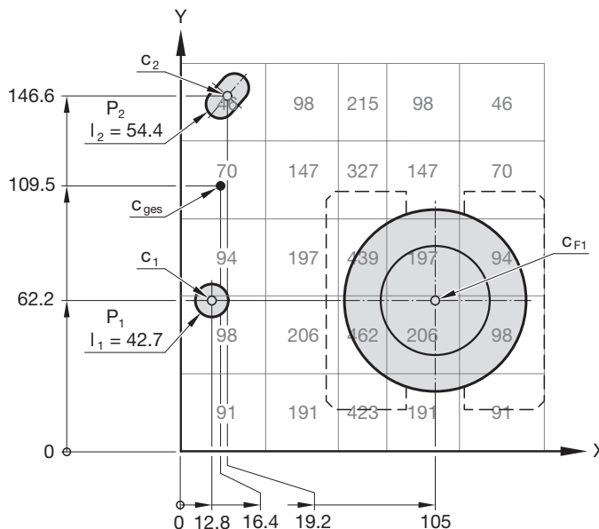
Immagine 24: Modello di foro eccentrico con molla di compensazione
