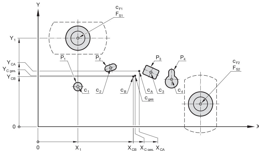
Immagine 9: Modello di foro con molla a gas
