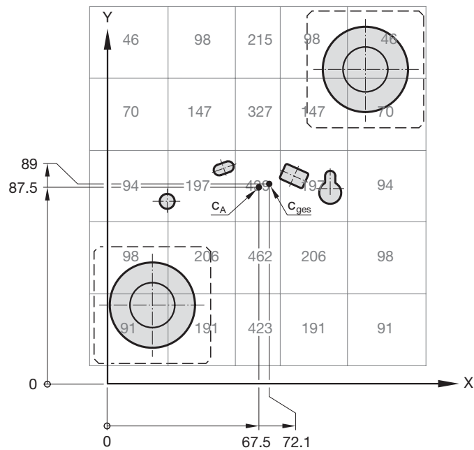
Immagine 17: Modello di foro con piastra raschiatore e diagramma delle forze
