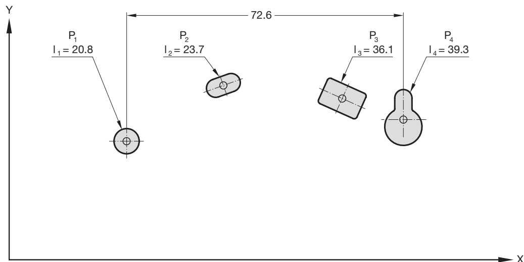
Immagine 13: Modello di foro con stima delle misure
