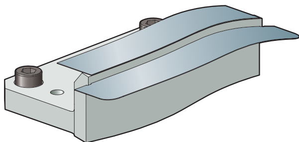
Immagine 18: Lama con affilatura parallela
