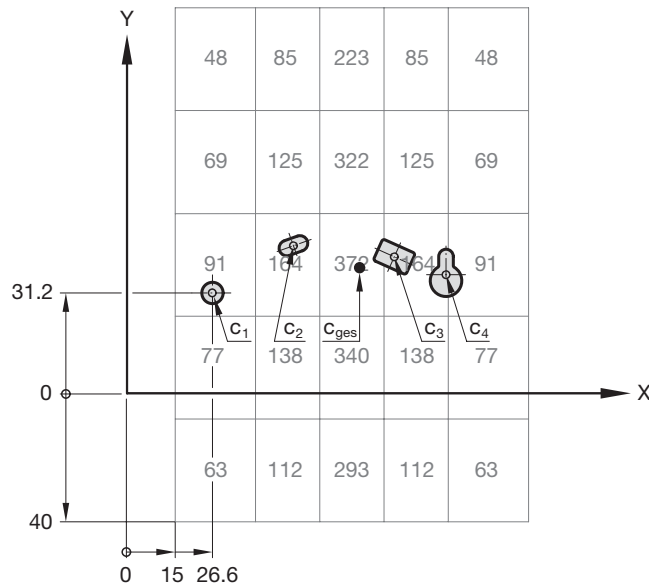
Immagine 15: Modello di foro con diagramma delle forze
