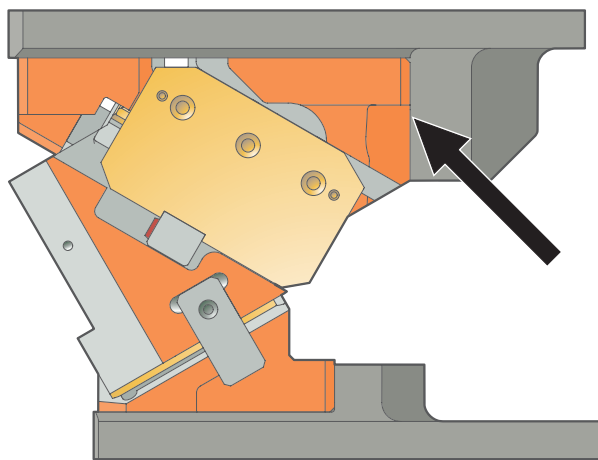
Immagine 1: Basamento del cursore con spallamento completo
