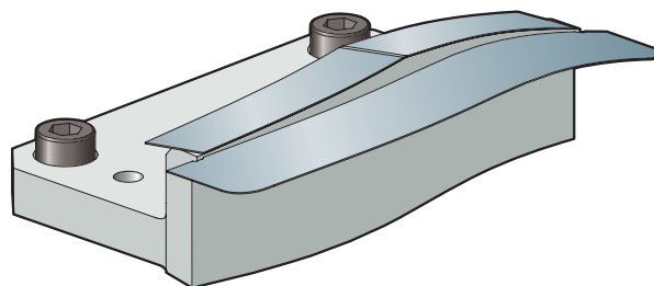
Immagine 19: Lama con affilatura a tetto
