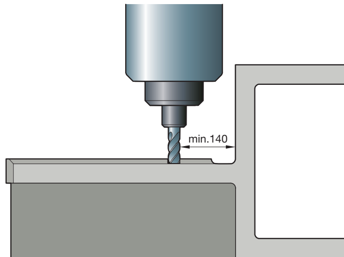
Immagine 4: Spazio libero mandrino di fresatura
