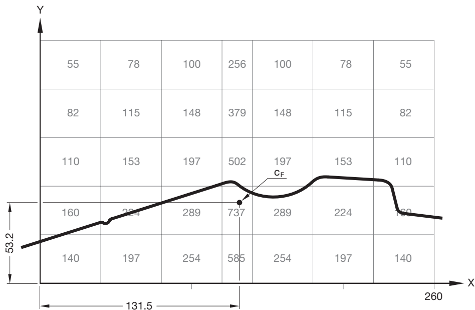
Immagine 12: Contorno di taglio con diagramma delle forze
