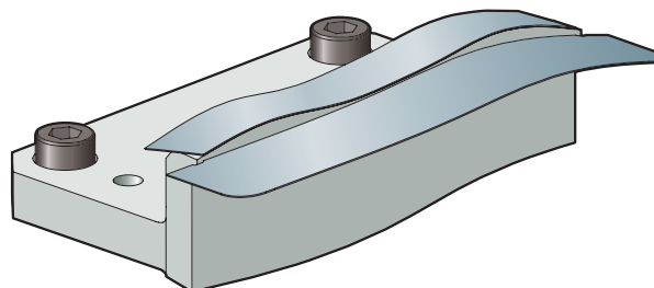
Immagine 21: Lama con affilatura a onda
