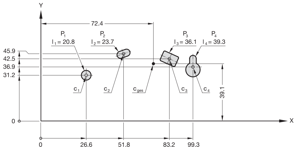
Immagine 14: Modello di foro con baricentri singoli
