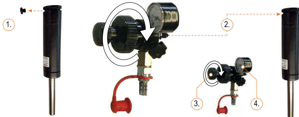
Fig. 2-2 Resortes de presión de gas con abertura de llenado lateral
