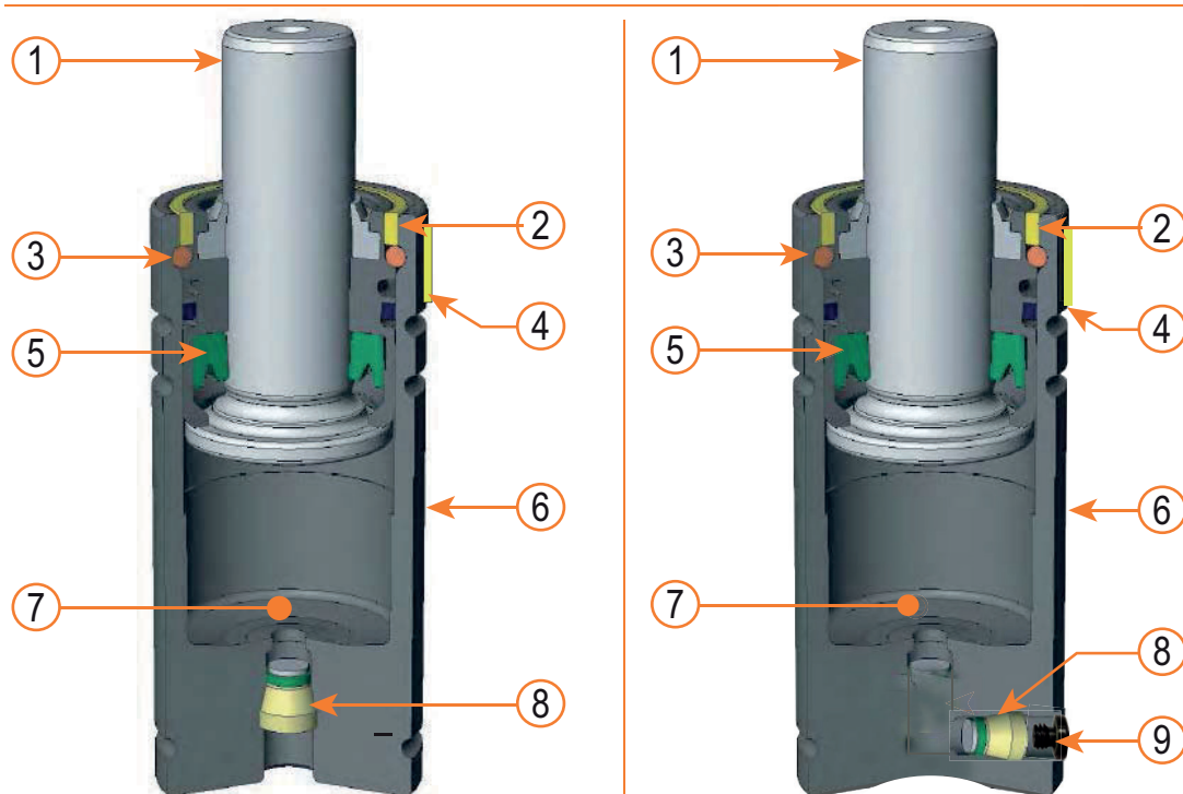
Fig. 2-5 Partes integrantes del resorte de presión de gas
