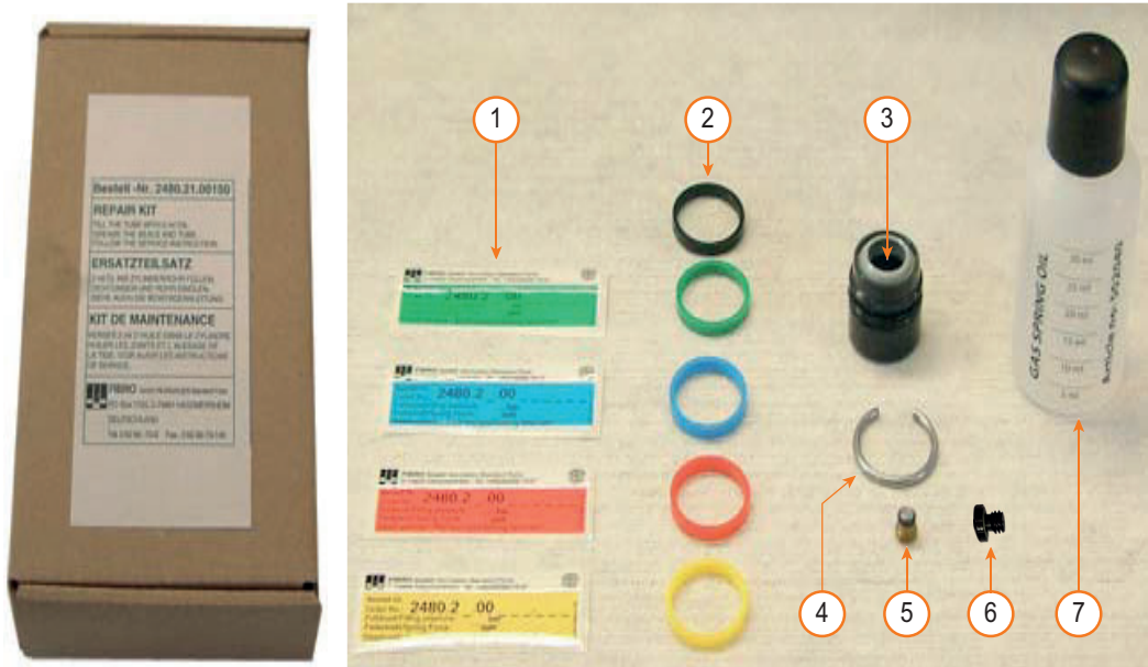
Fig. 2-6 Juego de piezas de repuesto del resorte de presión de gas 2480.2x./3x.
