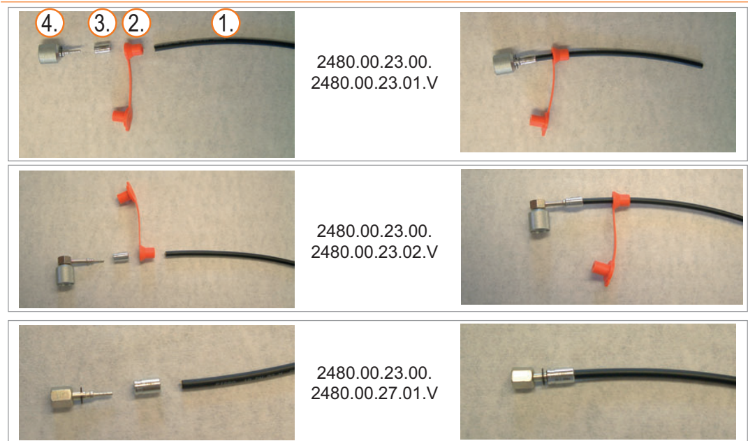
Fig. 5-4 Préparation d'un flexible
