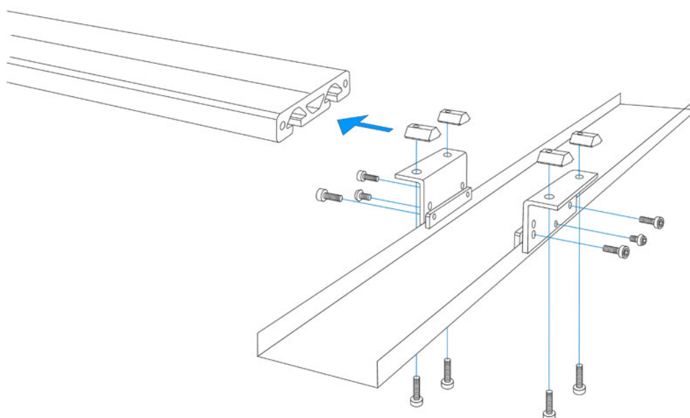
Fig. 5-19 Fissaggio canalina sospeso sulla barra profilata
