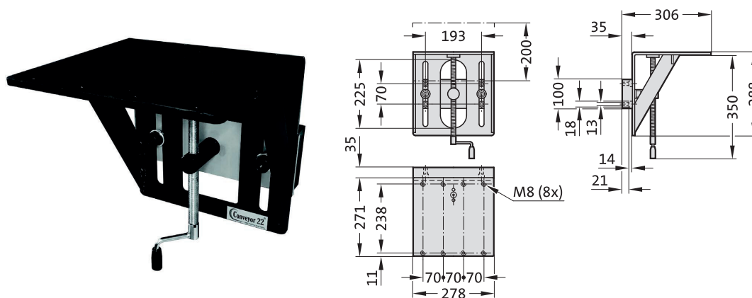
Fig. 5-11 Staffa di montaggio regolabile in altezza per il montaggio del convogliatore
