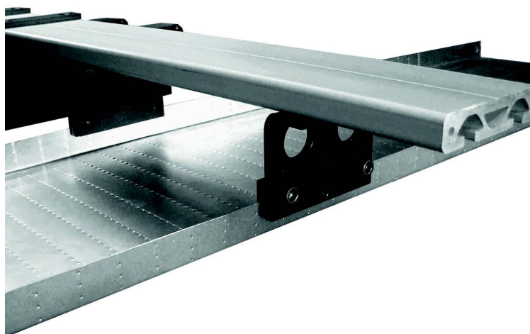
Fig. 5-8 Kit di montaggio fissaggio canalina sospeso
