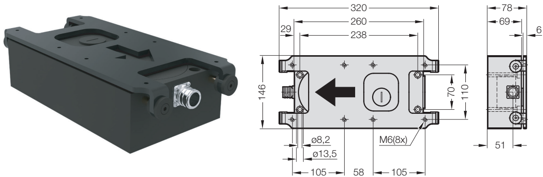
Fig. 3-5 Dimensioni convogliatore elettrico BLACK LINE ULTRA
