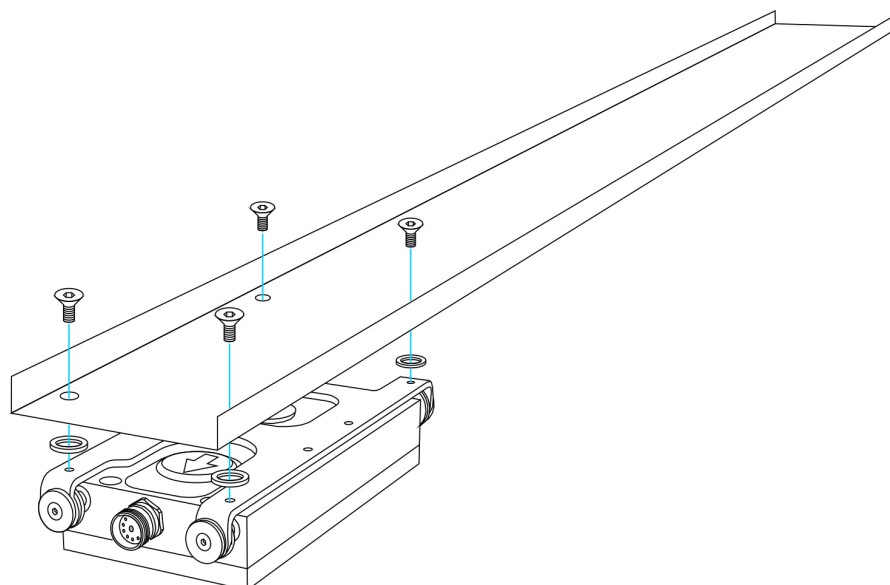
Fig. 5-14 Montare la canalina singola
