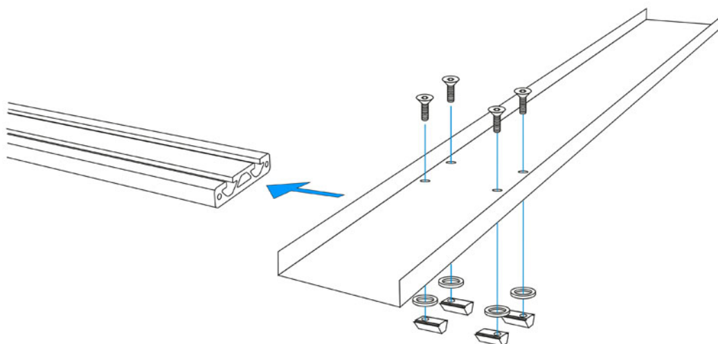
Fig. 5-17 Fissaggio della canalina con dadi scorrevoli
