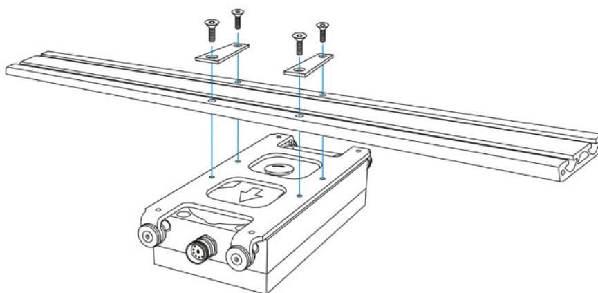
Fig. 5-16 Montare la barra profilata con le barre di fissaggio.
