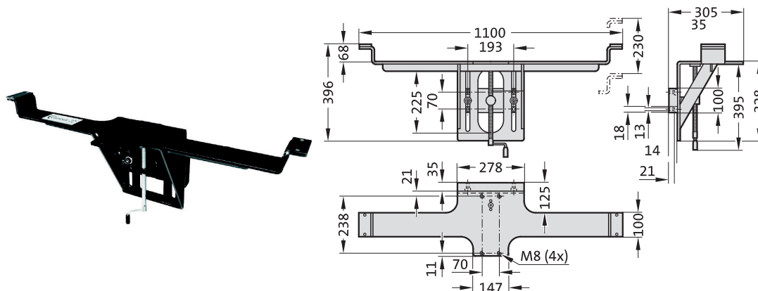
Rys. 5-12 Kątownik montażowy z regulacją wysokości do montażu belki profilowej
