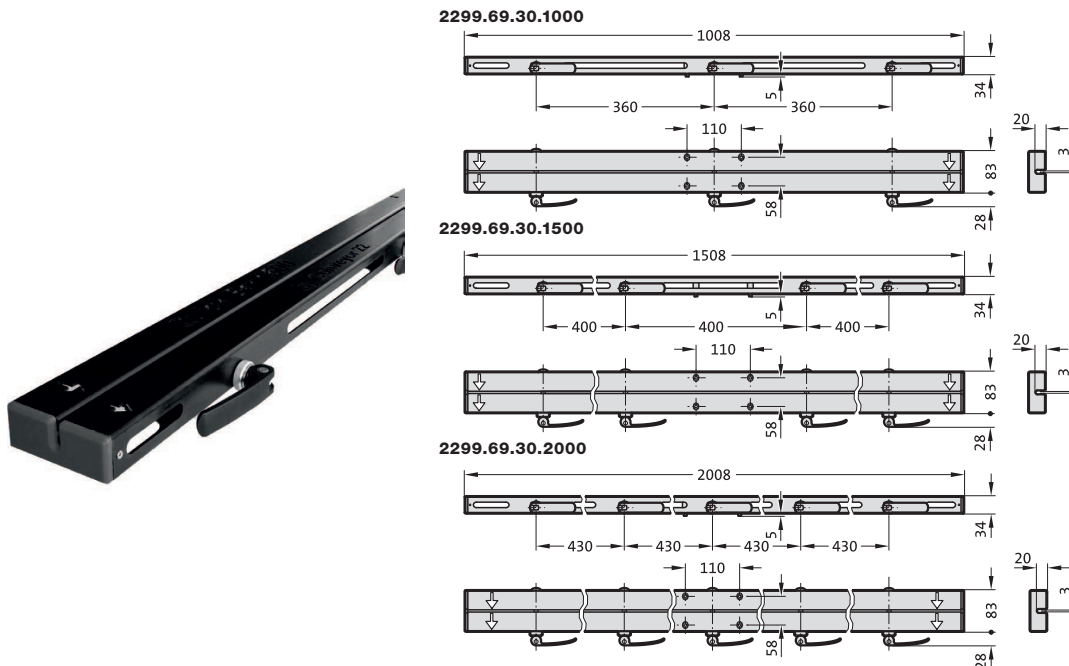
Rys. 5-10 Szyny zaciskowe
