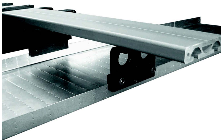
Rys. 5-8 Zestaw montażowy mocowania rynny na wisząco
