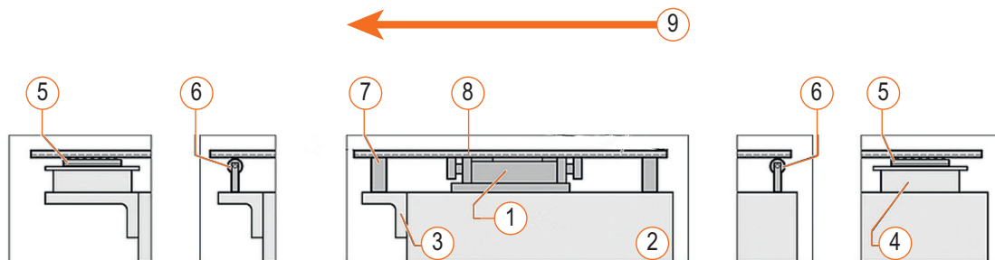
Rys. 5-20 Podparcia rynny
