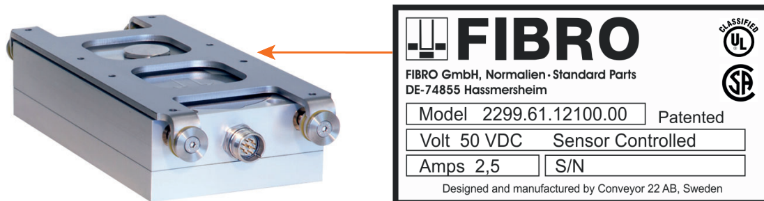
Abb. 3-5 Typenschild
