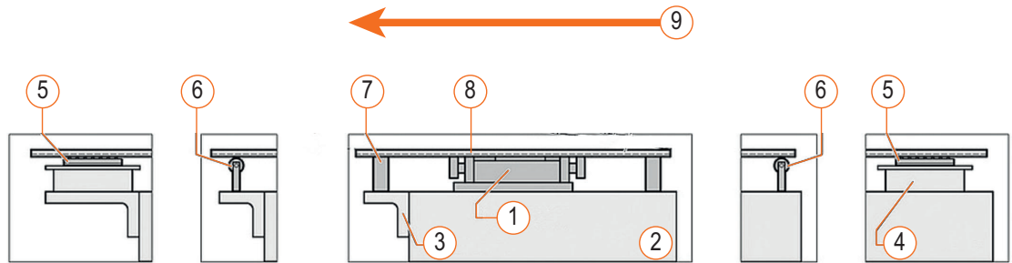
Abb. 5-6 Rinnenunterstützungen
