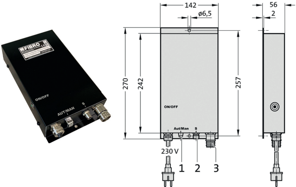
Fig. 3-2 Dimensions de l'unité de commande BLACK LINE
