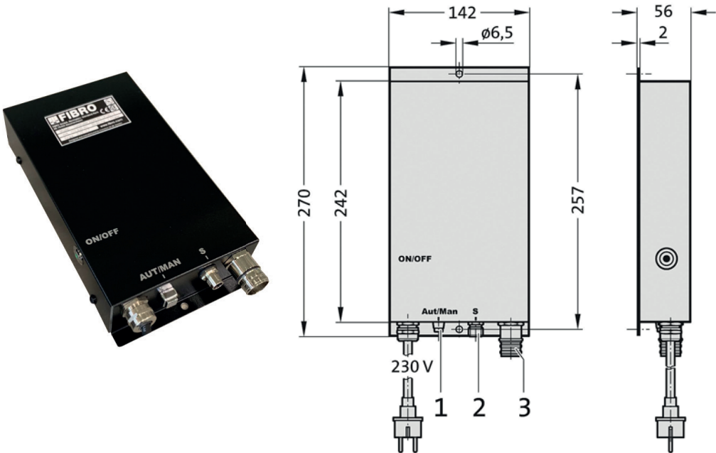
Abb. 3-2 Abmessungen Steuereinheit BLACK LINE
