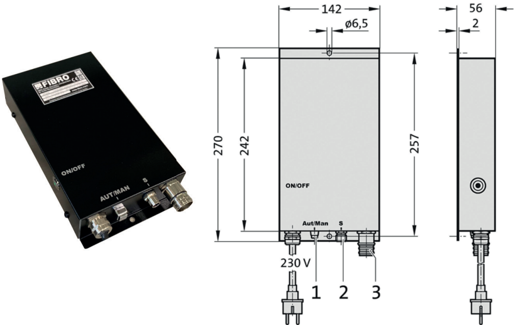
Fig. 3-2 Dimensiones unidad de control BLACK LINE
