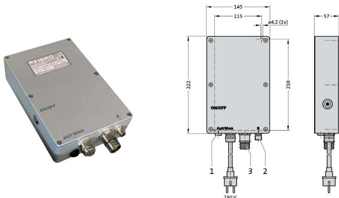
Fig. 3-2 Dimensiones unidad de control CLEAN LINE
