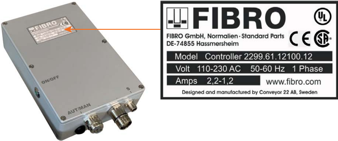
Fig. 3-3 Placa de características
