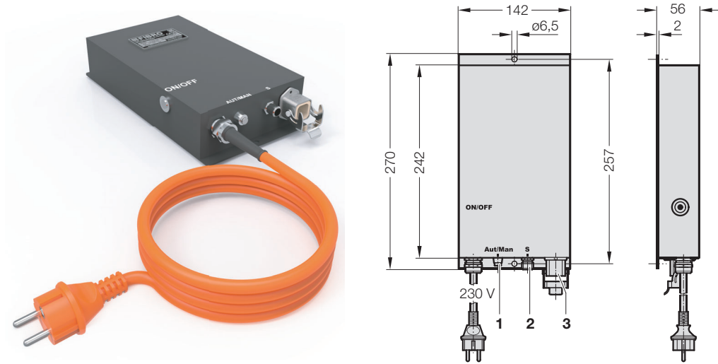
Abb. 3-2 Abmessungen Steuereinheit BLACK LINE EX
