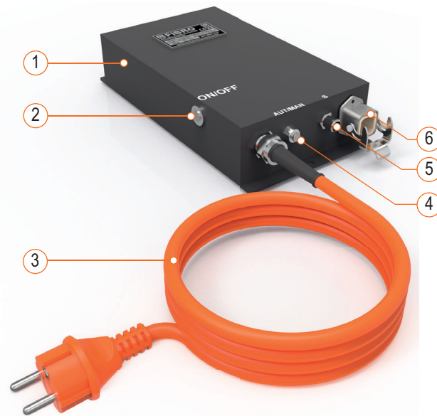
Abb. 3-1 Komponenten der Steuereinheit BLACK LINE EX
