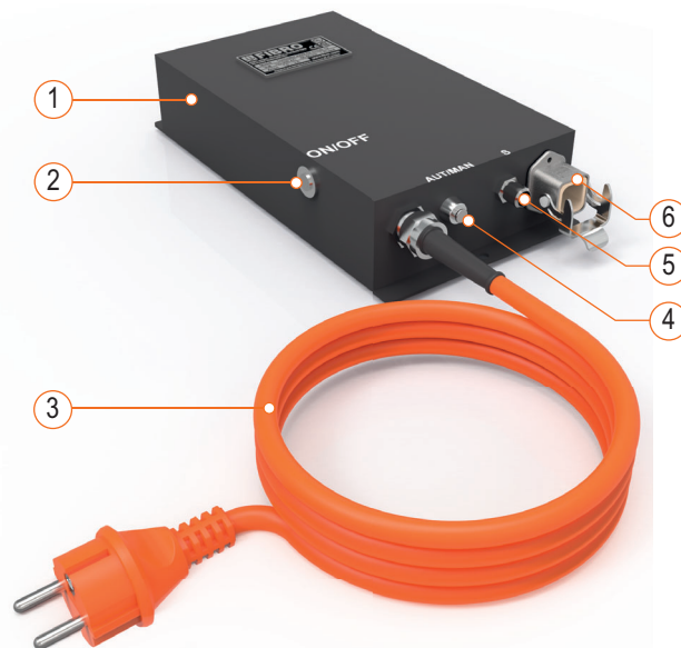
Fig. 3-1 Componenti della centralina di controllo BLACK LINE EX
