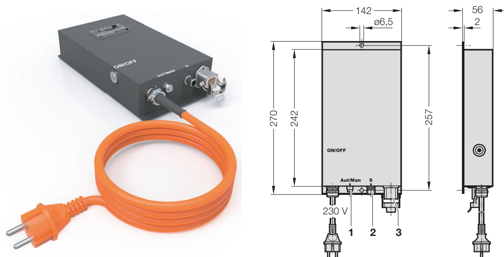
Fig. 3-2 Dimensioni centralina di controllo BLACK LINE EX
