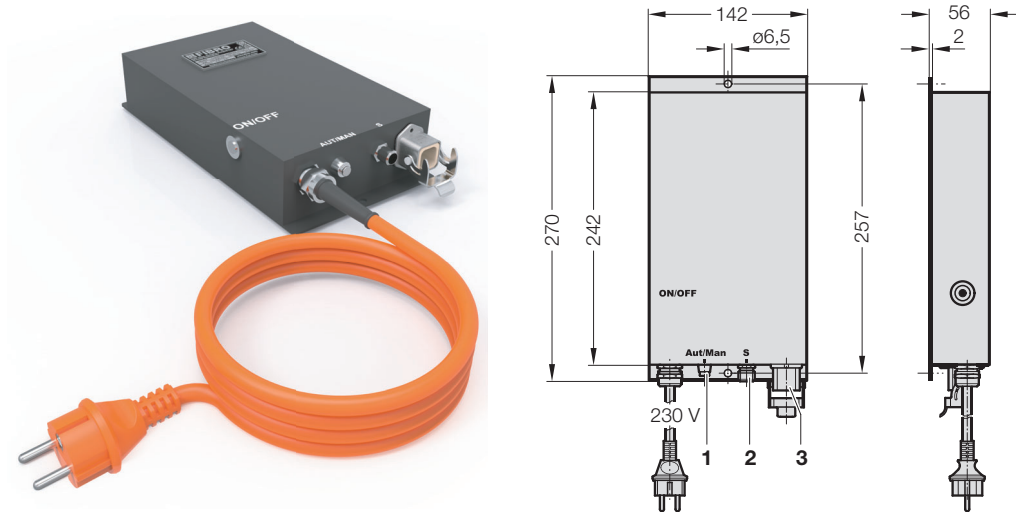
Rys. 3-2 Wymiary jednostki sterującej BLACK LINE EX
