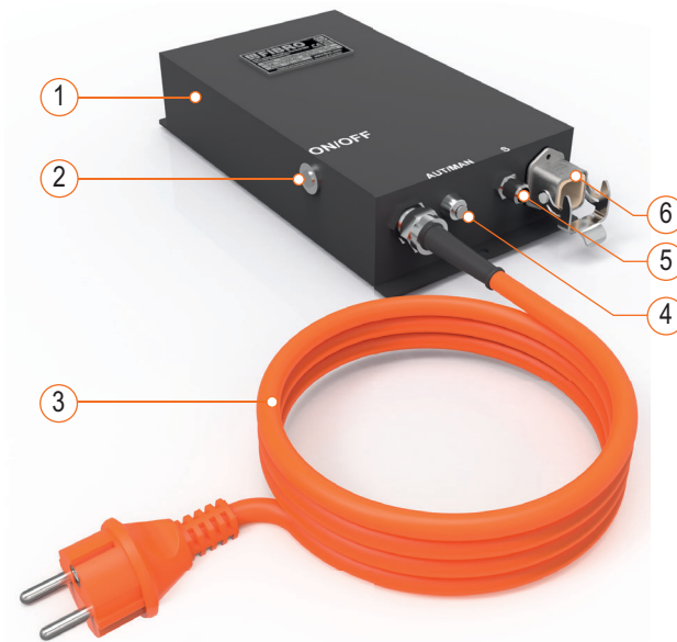
Rys. 3-1 Komponenty jednostki sterującej BLACK LINE EX
