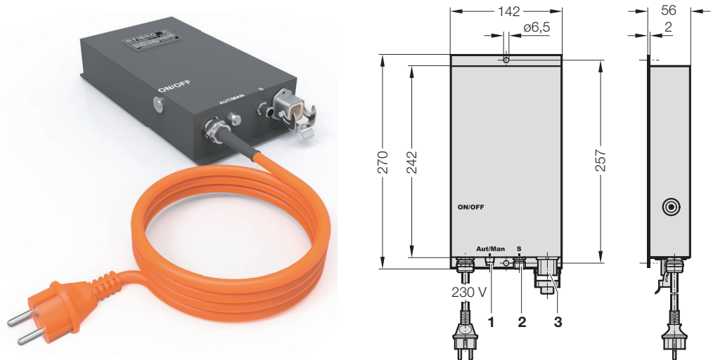
Fig. 3-2 Dimensiones unidad de control BLACK LINE EX
