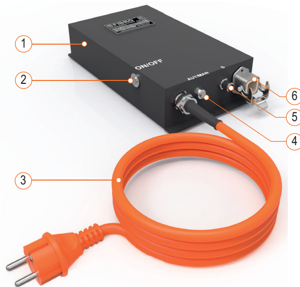
Fig. 3-1 Componentes de la unidad de control BLACK LINE EX
