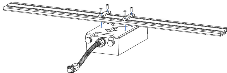
Abb. 5-16 Profilbalken mit Halteleisten montieren
