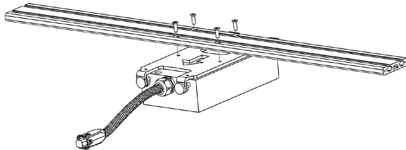
Abb. 5-15 Profilbalken mit Spezialschrauben montieren
