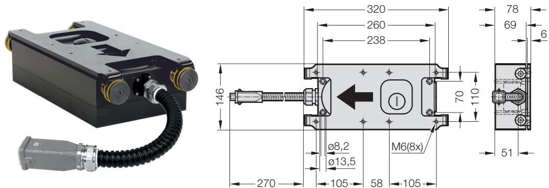
Abb. 3-4 Abmessungen Transporter, elektrisch BLACK LINE ULTRA EX
