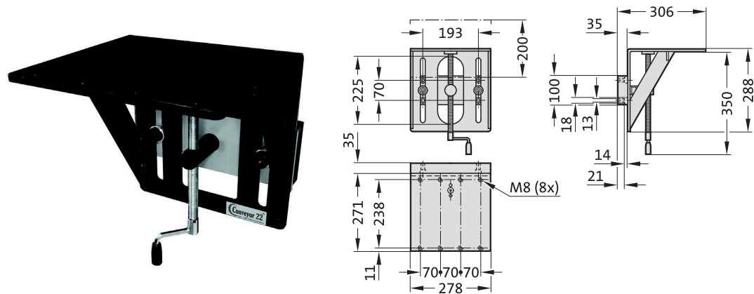
Abb. 5-11 Montagewinkel höhenverstellbar für Transportermontage
