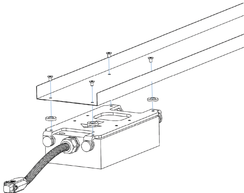
Abb. 5-14 Einzelrinne montieren
