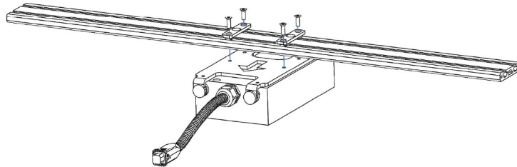
Fig. 5-16 Montare la barra profilata con le barre di fissaggio.
