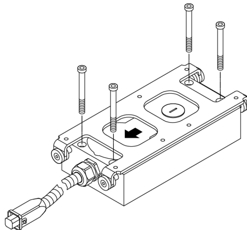
Fig. 5-13 Montaggio del convogliatore elettrico
