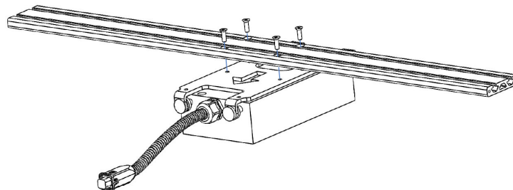
Fig. 5-15 Montare la barra profilata con le viti speciali.
