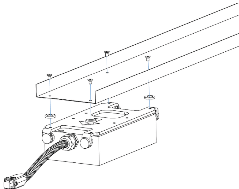
Fig. 5-14 Montare la canalina singola
