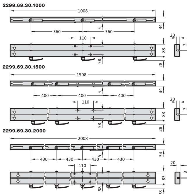
Rys. 5-10 Szyny zaciskowe
