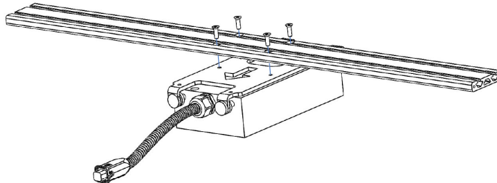
Rys. 5-15 Montaż belki profilowej specjalnymi śrubami
