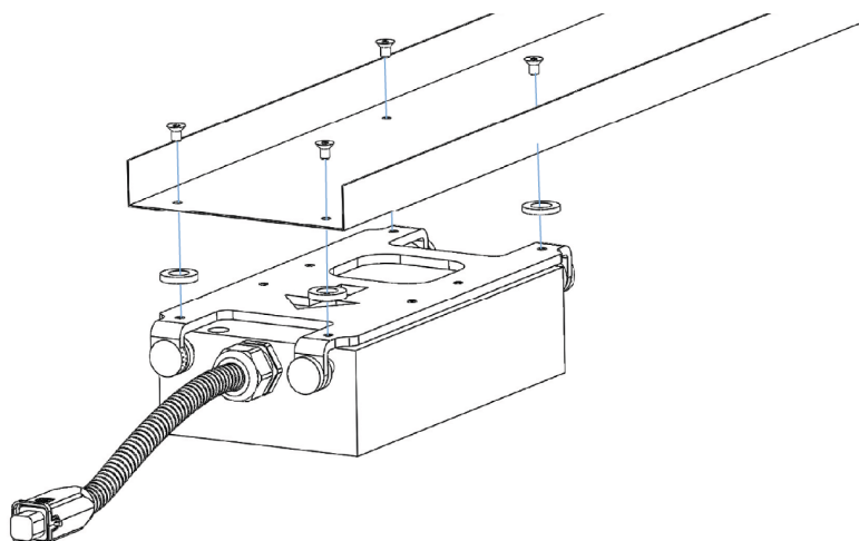
Rys. 5-14 Montaż rynny pojedynczej
