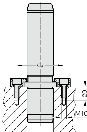
Příklad montáže
