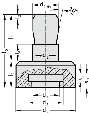
212.16. Attacco per codolo di accoppiamento
