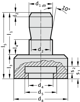
212.16. Perno de acoplamiento con guía
