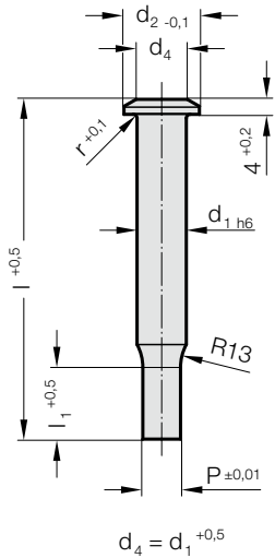
2210. Schneidstempel, abgesetzt, Rund, ~DIN 9844
