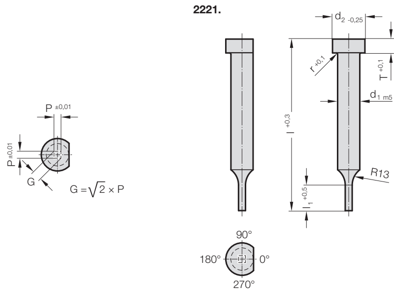
2221. Punzone da tranciatura, a diametro ridotto, quadrato, ISO 8020
