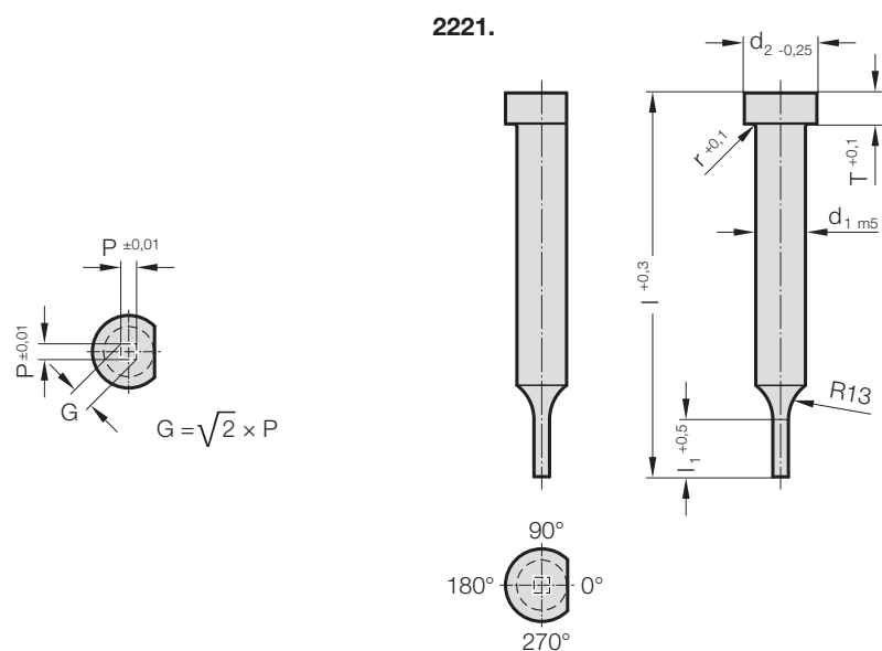
2221. Punzón de corte, con mecha, cuadrado, ISO 8020
