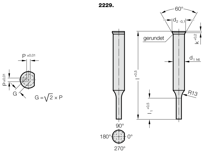
2229. Schneidstempel, abgesetzt, Quadrat, ~ DIN 9861
