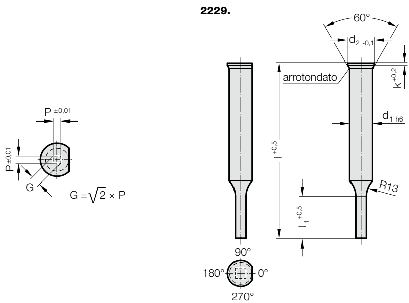
2229. Punzone da tranciatura, a diametro ridotto, quadrato, ~ DIN 9861
