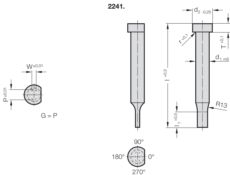
2241. Střížník, osazené, Oválný otvor, ISO 8020
