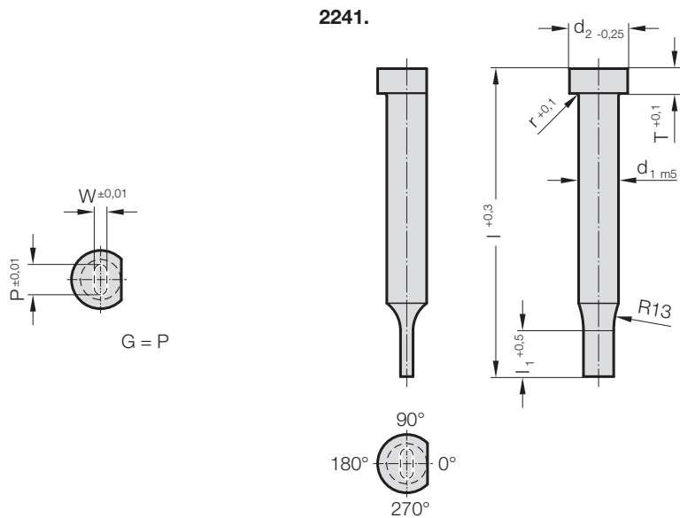
2241. Punzone da tranciatura, a diametro ridotto, asola, ISO 8020
