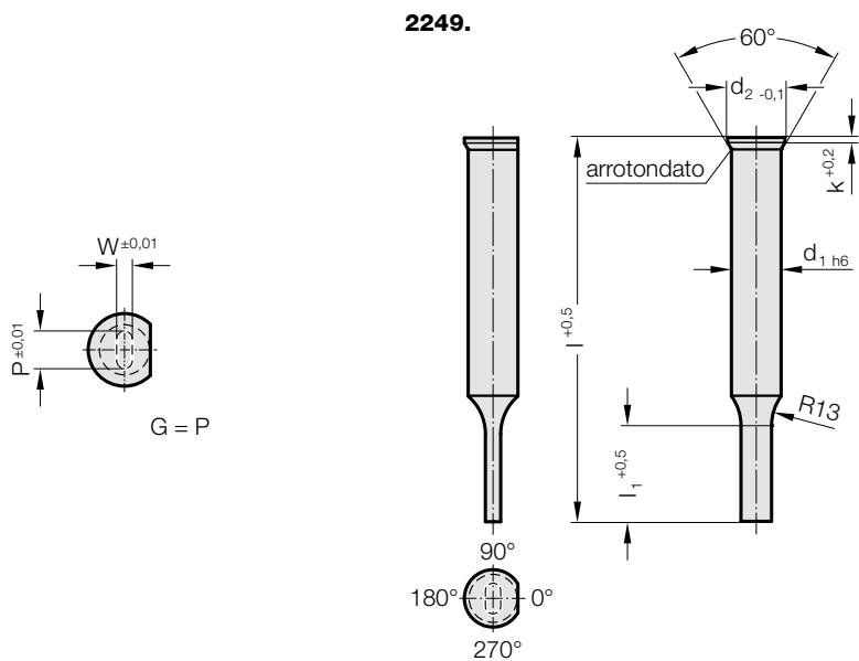
2249. Punzone da tranciatura, a diametro ridotto, asola, ~ DIN 9861
