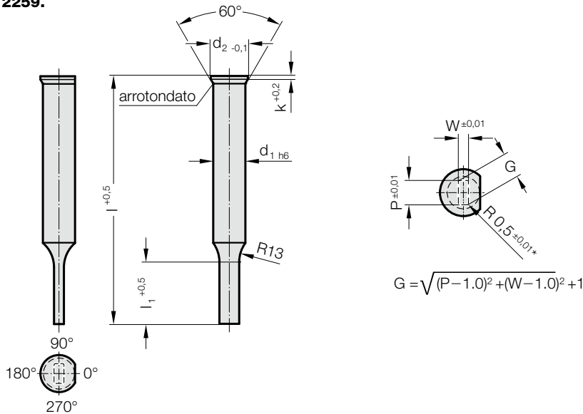
2259. Punzone da tranciatura, a diametro ridotto, rettangolo con angoli raggiati, ~DIN 9861
