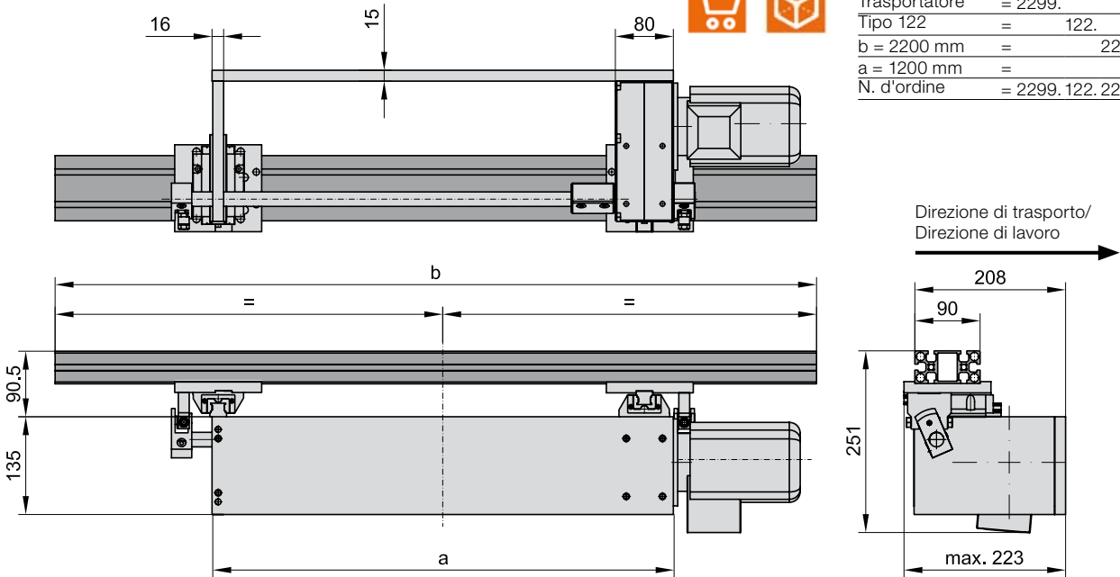
2299.122. Posizione riduttore orizzontale, 2 slitte, con profilo e supporto
