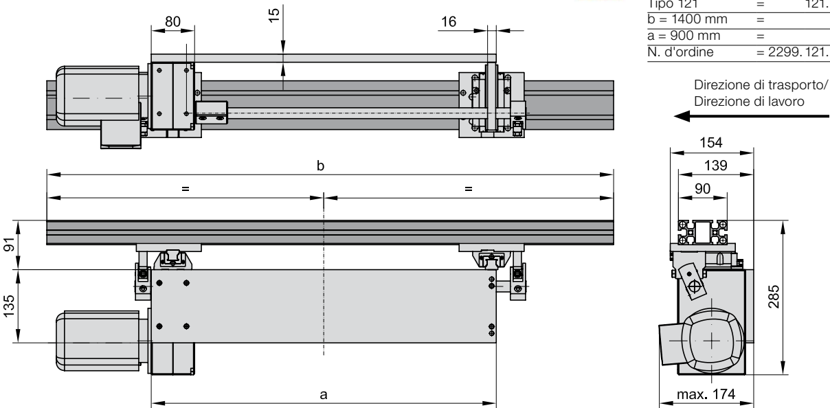
2299.121. Posizione riduttore verticale, 2 slitte, con profilo e supporto
