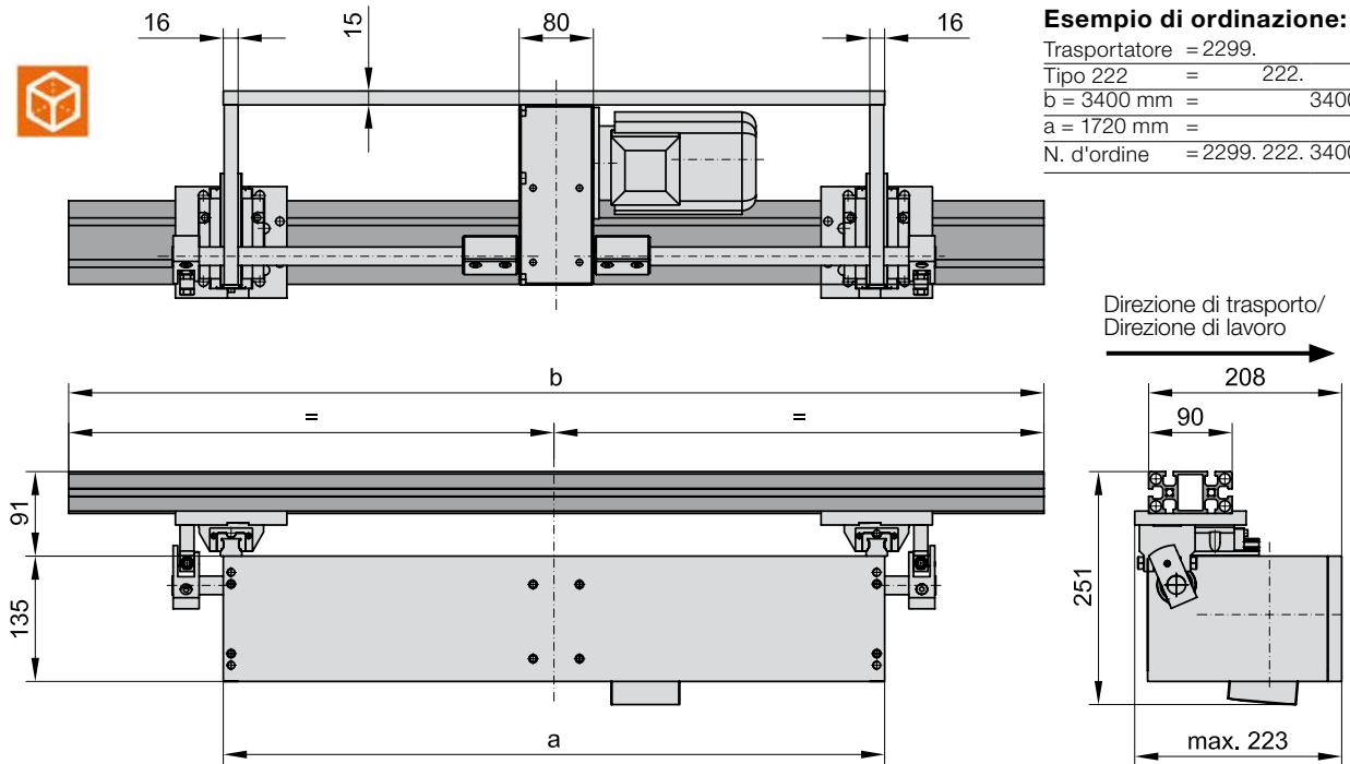
2299.222. Posizione riduttore orizzontale centrale, 2 slitte, con profilo e supporto
