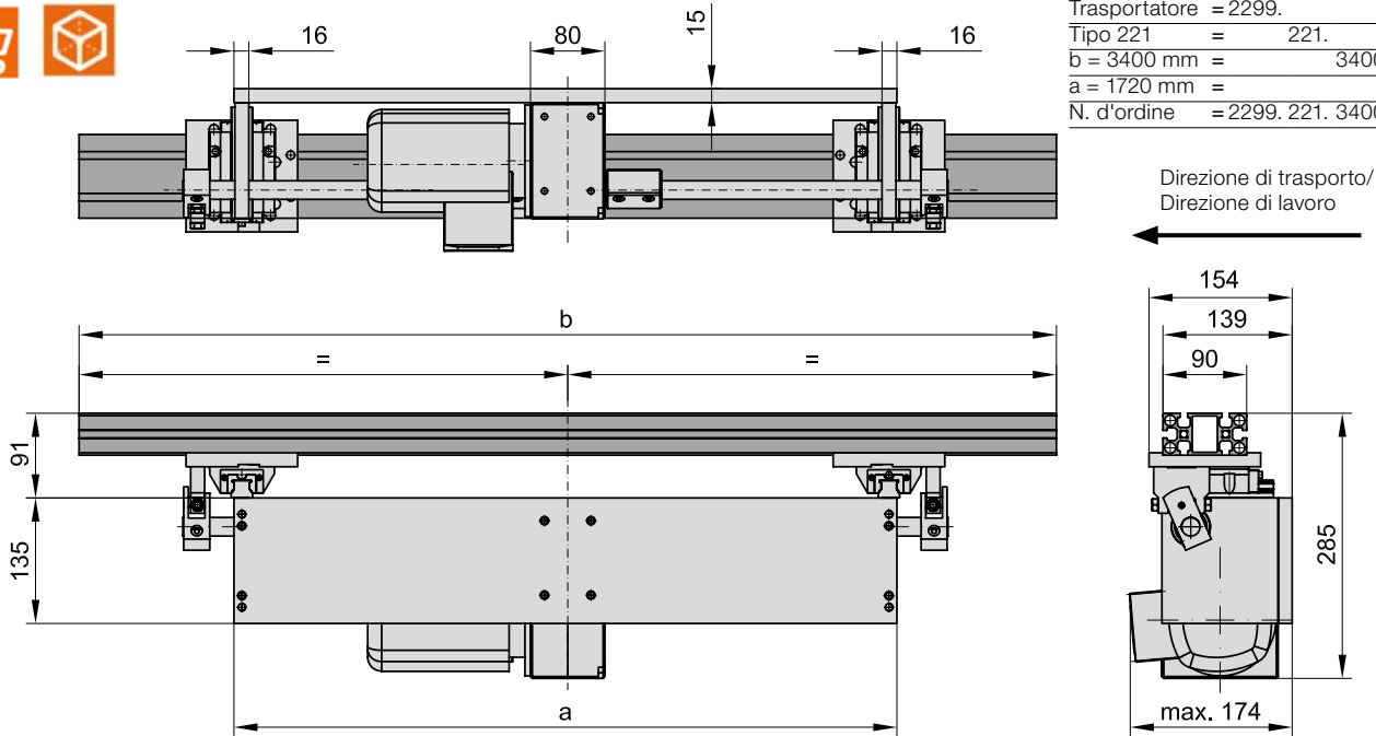
2299.221. Posizione riduttore verticale centrale, 2 slitte, con profilo e supporto
