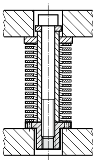
Příklad montáže
