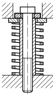
Przykład zabudowy
