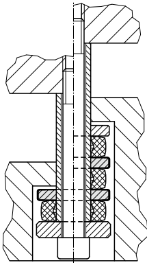
Esempio di montaggio
