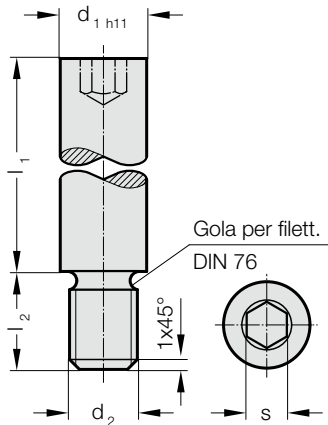
244.5. Spina di guida
