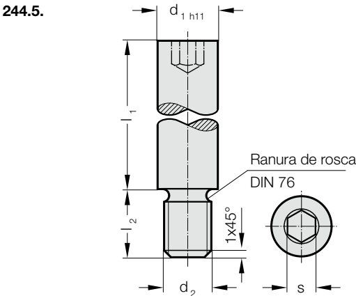
244.5. Perno de guía
