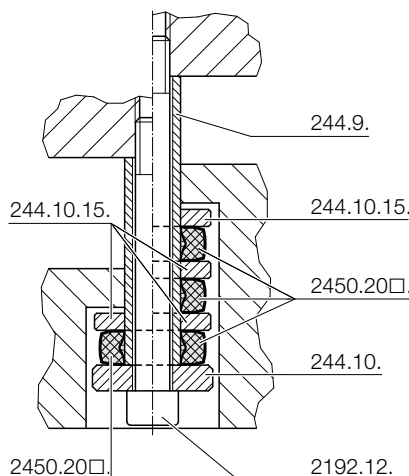
Příklad montáže
