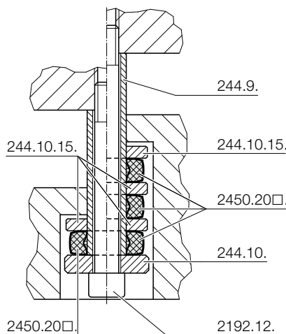
Przykład zabudowy
