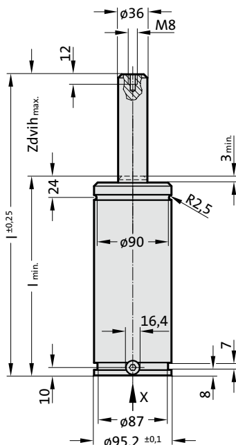
Pohled X - Plynová pružina
