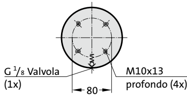
Vista in direzione X - Molla a gas
