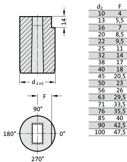
Verdrehsicherung 5 (5)
