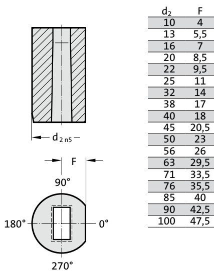
Verdrehsicherung 4 (4)
