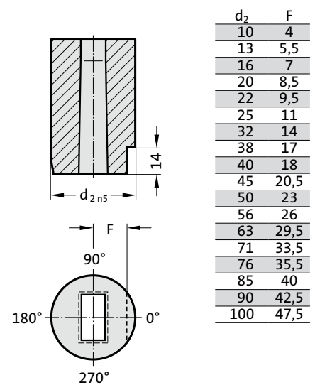
Verdrehsicherung 6 (6)
