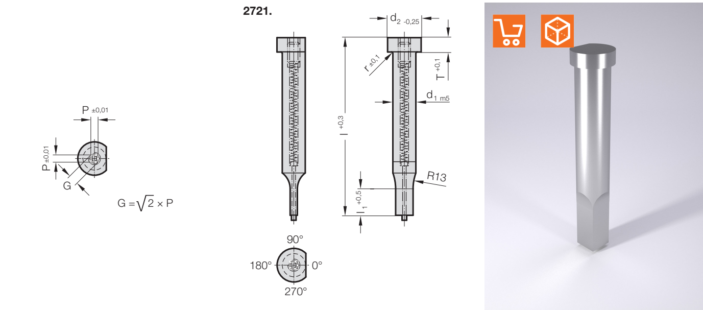
2721. Stempel ISO 8020 z odsadzeniem i odklejaczem (kwadrat)
