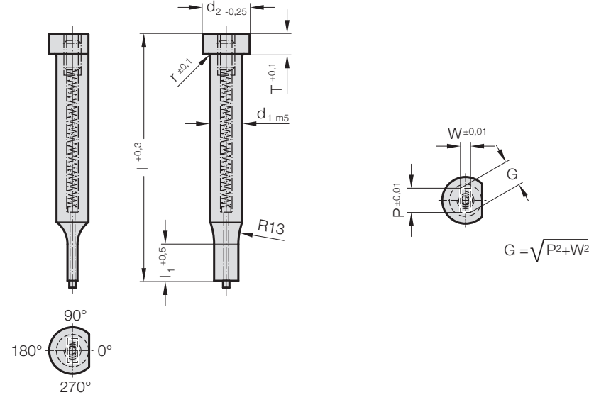
2731. Punzone da tranciatura, a diametro ridotto, rettangolo, con spina di espulsione, ISO 8020
